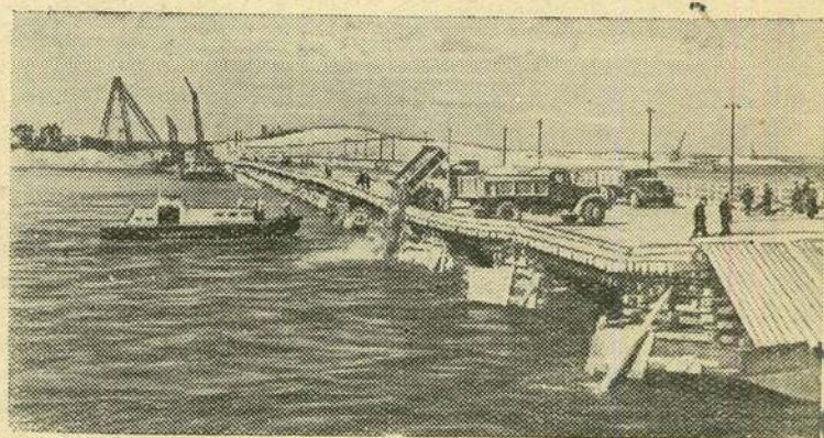
Горьковская область. Для перекрытия русла Волги на строительстве Горьковской гидроэлектростанции сооружен понтоновый мост шириной в 20 метров и длиной в 300 метров, с которого автосамосвалы сбрасывают камень.
