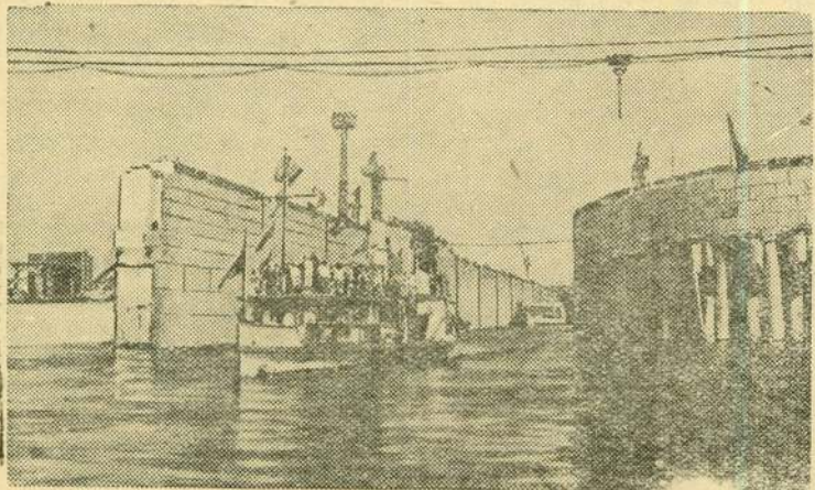
На строительстве Куйбышевской гидроэлектростанции со- стоится пуск нижних судоходных шлюзов. НА СНИМКЕ: выход первых судов из камеры шлюза. Фото А. Батанова. Фотохроника ТАСС.
