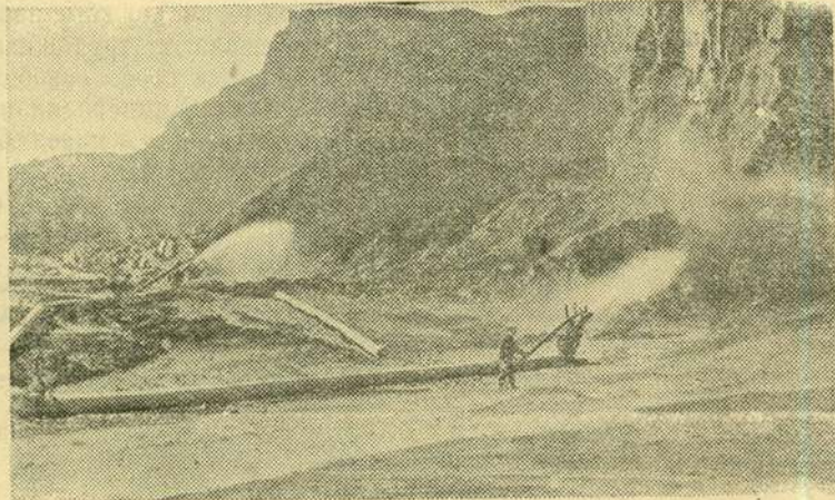
Челябинская область. На Батуринском угольном разрезе № 3—4 треста «Коркинуголь» наряду с экскаваторными работами широко применяется гидромеханизация на вскрыше и добыче угля. Этот метод комплексной механизации позволяет разрабатывать и транспортировать породу и уголь, обогащать его и убирать отходы в отвал. Гидромеханизаторы Батуринского разреза систематически перевыполняют план.
