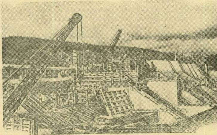
Башкирская АССР. На строительстве Уфимской ГЭС. НА СНИМКЕ: бетонные работы на строительстве шлюза. Фото Г. Ефимова. Фотохроника ТАСС.
