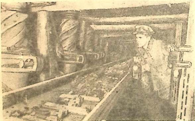
Сталинская область. Шахта имени инженера Абакумова — одна из крупнейших в Донбассе. В лавах введена металлическая органическая крепь. Ее применение значительно сокращает трудоемкость работ, способствует увеличению производительности угольных комбайнов.
