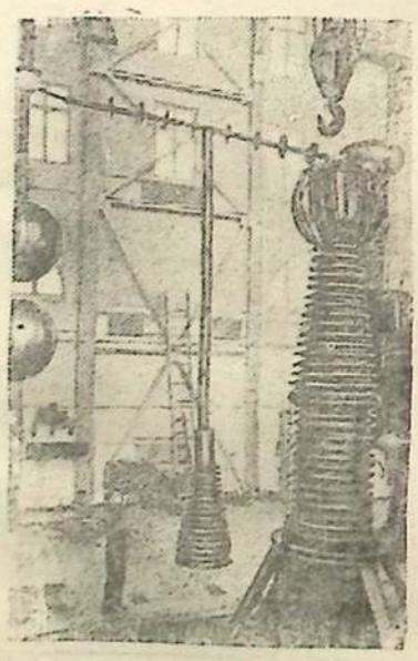
На московском заводе „Изолятор“ построена и пущена в эксплуатацию станция для испытательных высоковольтных изоляторов линий электропередач и трансформаторов.
